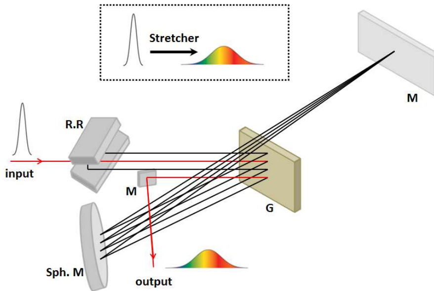
Σχήμα 2.4: Σχηματική αναπαράσταση του Stretcher. Όπου R.R περισκόπιο για κατακόρυφο ανέβασμα της δέσμης, G φράγμα περίθλασης, Sph.M. σφαιρικό κάτοπτρο μεγάλης διαμέτρου, M επίπεδα κάτοπτρα υψηλής ανακλαστικότητας στα 800 nm.
