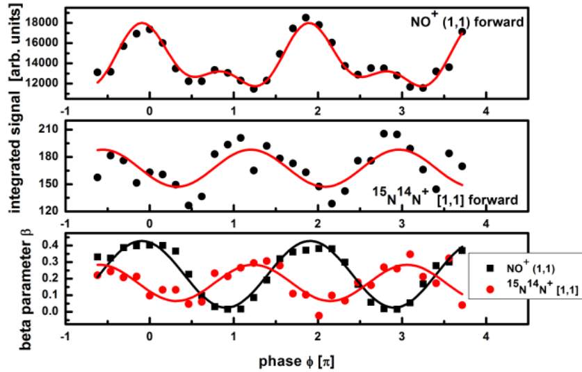
Σχήμα 3.19: Η εξάρτηση του ολοκληρώματος της forward συνιστώσας των σημάτων \text{NO}^+(1,1) και ^{15}\text{N}^{14}\text{N}^+[1,1] και οι αντίστοιχες καμπύλες ασυμετρίας \beta .
