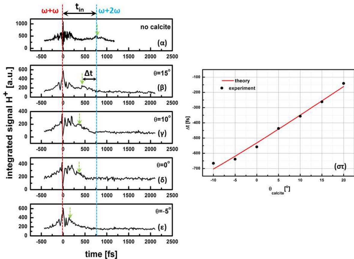
Σχήμα Β'2: Το ολοκλήρωμα του σήματος του H^+ ως συνάρτηση του χρόνου καθυστέρησης της δέσμης probe για (α) απουσία των κρυστάλλων calcite 1,2 και (β)-(ε) επιλεγμένες γωνίες στροφής του κρυστάλλου calcite 2. Η χρονική επικάλυψη της δέσμης \omega -probe και 2\omega -rump σημειώνεται με πράσινο βέλος. Όσο αυξάνει η γωνία στροφής του κρυστάλλου calcite 2 η δύο επικαλύψεις \omega + \omega και \omega + 2\omega τείνουν να συμπέσουν στον χρόνο. (στ) Το διάγραμμα της διαφοράς χρόνου \Delta t ως συνάρτηση της γωνίας \theta του calcite 2. Με μαύρους κύκλους συμβολίζονται τα πειραματικά σημεία ενώ η κόκκινη συμπαγής γραμμή είναι η αντίστοιχη θεωρητική καμπύλη.
