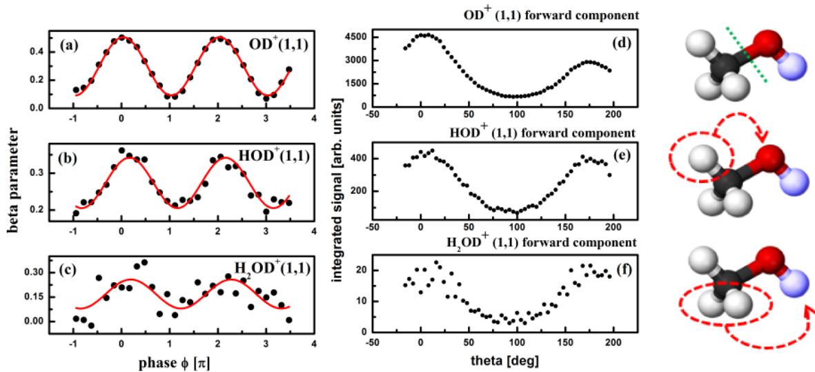
Σχήμα 4.5: (a)-(c) Οι καμπύλες ασυμμετρίας \beta των θραυσμάτων OD^+(1,1) , HOD^+(1,1) , H_2OD^+(1,1) μετά από ακτινοβολία της μεθανόλης CH_3OD με ασύμμετρο πεδίο laser \omega/2\omega έντασης I \simeq 6.6 \cdot 10^{14} \text{ W/cm}^2 και (d)-(f) οι αντίστοιχες γωνιακές κατανομές τους για σταθερή φάση \varphi = 0 . Τα πειραματικά δεδομένα αναπαριστώνται με σημεία, ενώ οι κόκκινες συμπαγείς γραμμές στα (a)-(c) είναι προσαρμογή με ημιτονοειδή συνάρτηση ( f(x) = A \sin(x - x_c) + bg ). Στο ίδιο σχήμα δίνονται και σχηματικές αναπαραστάσεις της μεταφοράς υδρογόνου.
