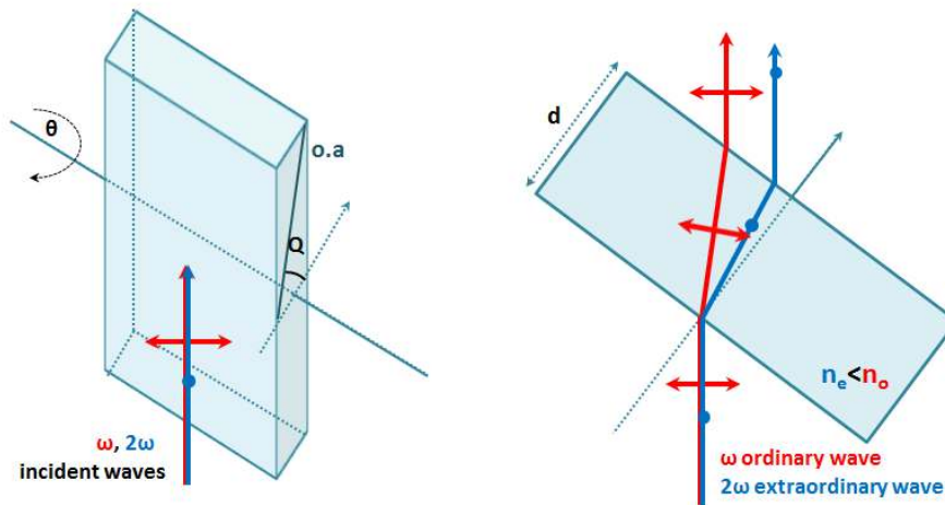
Σχήμα 2.8: Ο προσανατολισμός των κρυστάλλων ασβεστίτη. Όπως είναι φανερό ότι η τακτική ακτίνα είναι η θεμελιώδης συχνότητα \omega και η έκτακτη η δεύτερη αρμονική 2\omega . Όπου o.a. ο οπτικός άξονας του κρυστάλλου, Q η γωνία κοπής και d το πάχος του κρυστάλλου. Με \theta συμβολίζεται η γωνία στροφής του κρυστάλλου για να εισαχθεί έτσι η επιθυμητή καθυστέρηση στην θεμελιώδη συχνότητα. Οι οπτικοί δρόμοι των δύο συχνοτήτων μέσα στον κρύσταλλο.
