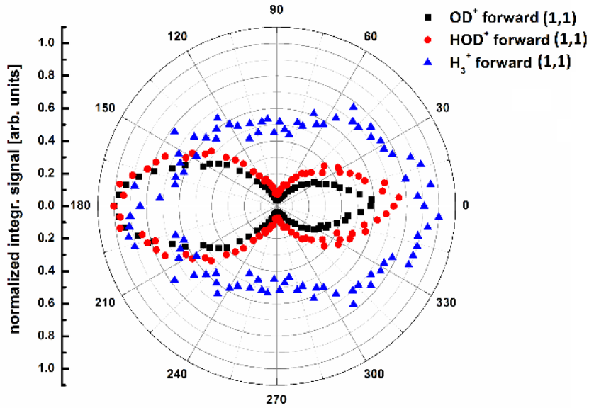
Σχήμα 4.8: Οι κανονικοποιημένες γωνιακές κατανομές των forward συνιστωσών των θραυσμάτων \text{OD}^+(1,1) , \text{HOD}^+(1,1) και \text{H}_3^+(1,1) μετά από ακτινοβολία της μεθανόλης \text{CH}_3\text{OD} με ασύμμετρο πεδίο laser \omega/2\omega για σταθερή φάση \varphi = \pi έντασης I \simeq 6.6 \cdot 10^{14} \text{ W/cm}^2 .
