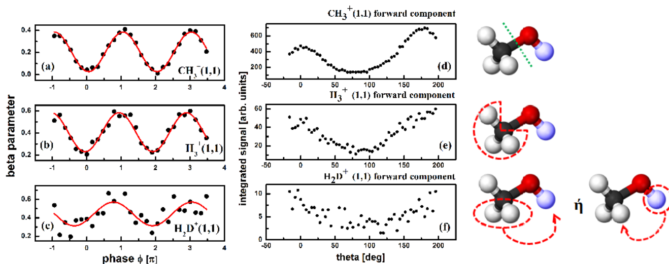
Σχήμα 4.6: (a)-(c) Οι καμπύλες ασυμμετρίας \beta των θραυσμάτων \text{CH}_3^+(1,1) , \text{H}_3^+(1,1) , \text{H}_2\text{D}^+(1,1) μετά από ακτινοβολία της μεθανόλης \text{CH}_3\text{OD} με ασύμμετρο πεδίο laser \omega/2\omega έντασης I \simeq 6.6 \cdot 10^{14} \text{ W/cm}^2 , όπου τα πειραματικά δεδομένα αναπαριστώνται με σημεία, ενώ οι κόκκινες συμπαγείς γραμμές είναι προσαρμογή με ημιτονοειδή συνάρτηση ( f(x) = A \sin(x - x_c) + bg ). (d)-(f) Οι γωνιακές κατανομές των θραυσμάτων \text{CH}_3^+(1,1) , \text{H}_3^+(1,1) , \text{H}_2\text{D}^+(1,1) για σταθερή φάση \varphi = 0 . Στο ίδιο σχήμα δίνονται και σχηματικές αναπαραστάσεις της μεταφοράς υδρογόνου.
