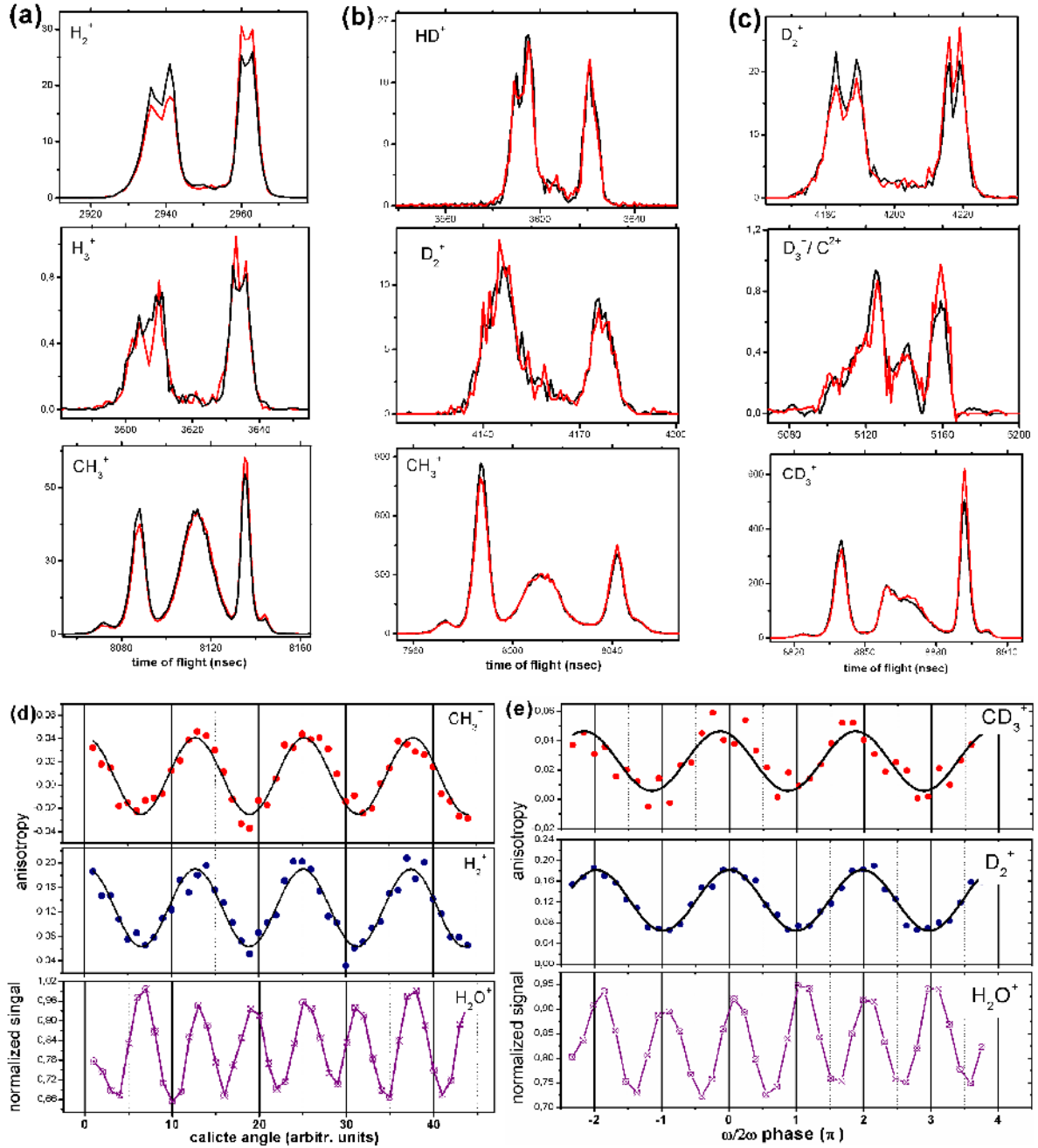
Σχήμα 4.13: (a)-(c) Μεγεθυμένες εικόνες διαφόρων ιοντικών θραυσμάτων του φάσματος μάζας των C_6H_5CH_3 , C_6D_5CH_3 και C_6D_5CD_3 αντίστοιχα, για ένταση I = 8 \cdot 10^{14} \text{ W/cm}^2 , όπου οι κορυφές μαύρης και κόκκινης γραμμή καταγράφηκαν σε σταθερή φάση \varphi = 0, \pi αντίστοιχα. (d),(e) Οι παράμετροι ασυμμετρίας \beta διαφόρων ιόντων των C_6H_5CH_3 και C_6D_5CD_3 αντίστοιχα, και το κανονικοποιημένο στην μονάδα ολοκλήρωμα του σήματος του νερού C_6H_5CH_3 , H_2O^+ σαν συνάρτηση της φάσης \varphi του πεδίου \omega/2\omega . Τα πειραματικά δεδομένα αναπαριστώνται με σημεία, ενώ οι συμπαγείς γραμμές είναι προσαρμογή με ημιτονοειδή συνάρτηση ( f(x) = A \sin(x - x_c) + bg ).
